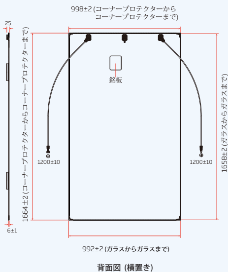
PVモジュールの寸法 (mm)
